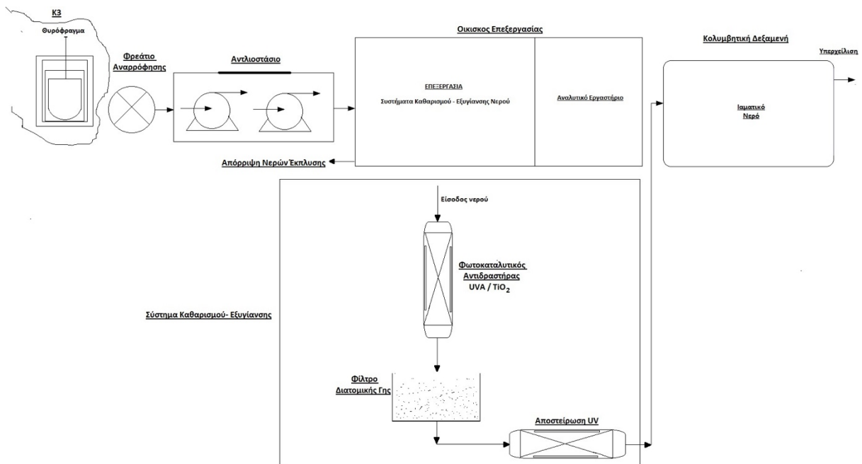
Διάγραμμα Ροής της Μονάδας Εξυγίανσης των Υδάτων (ΜΕΥ)
